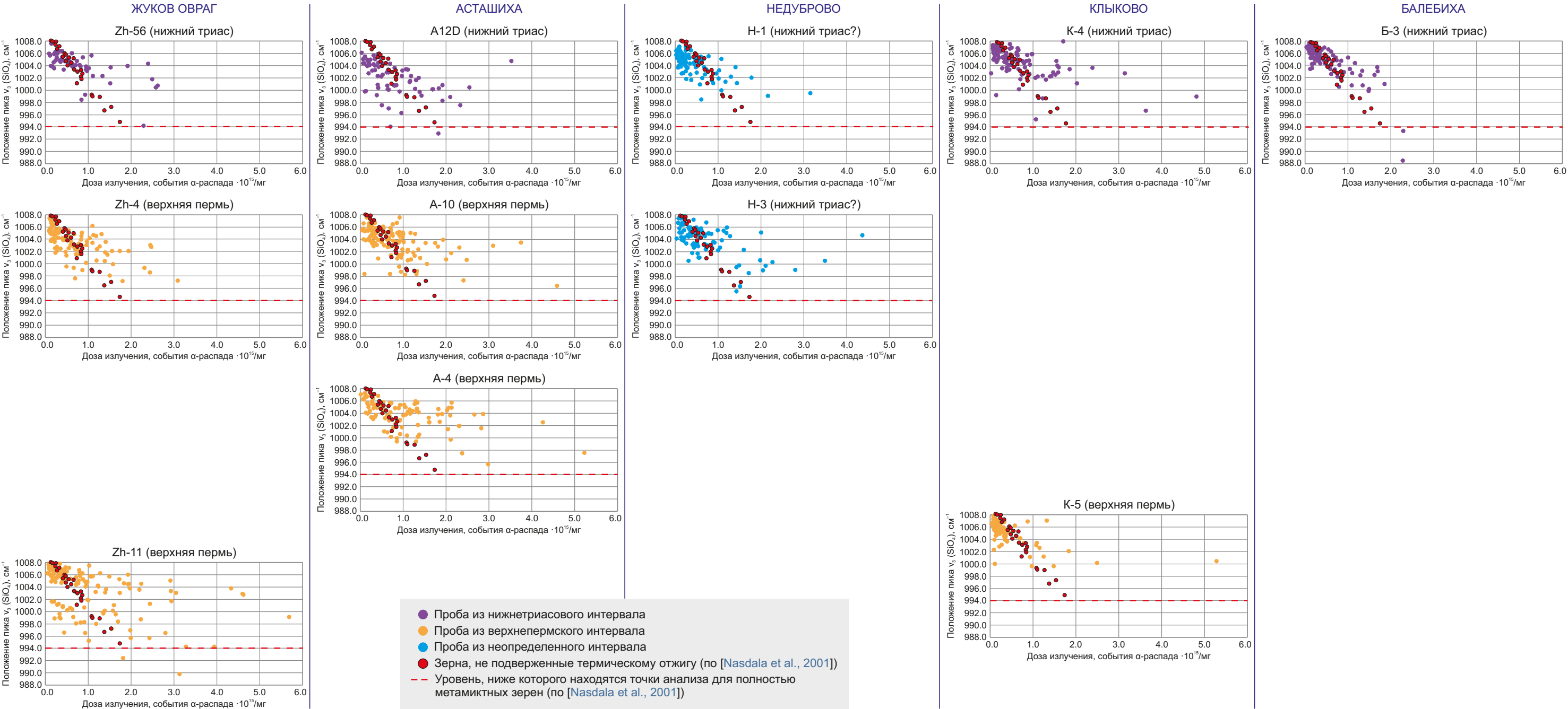
Графики зависимости положения рамановского пика \nu_3(\text{SiO}_4) от накопленной дозы альфа-излучения для изученных проб Relationships between \nu_3(\text{SiO}_4) Raman peak position and accumulated alpha-dose
