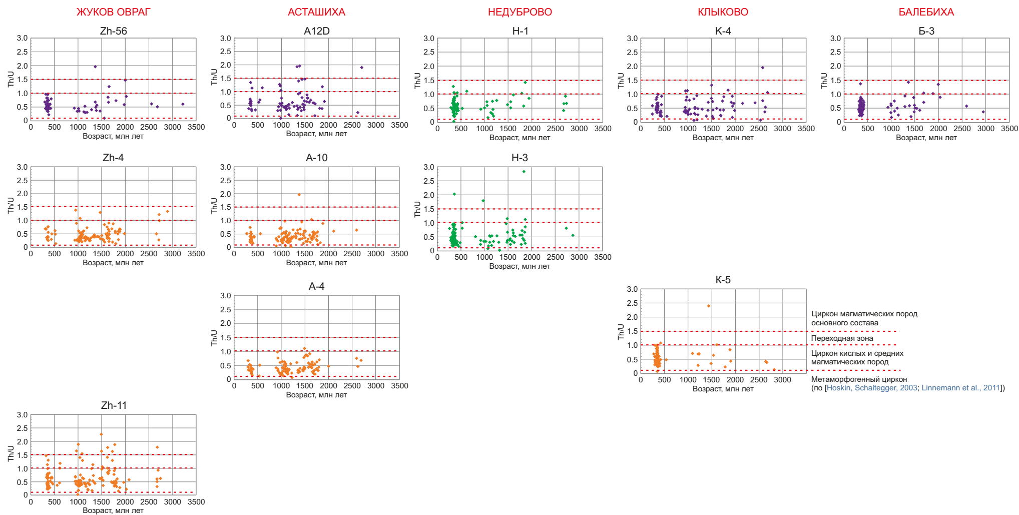
Графики зависимости Th/U отношений от возраста зерен обломочного циркона для изученных проб Relationships between Th/U ratios and detrital zircon U-Pb ages
