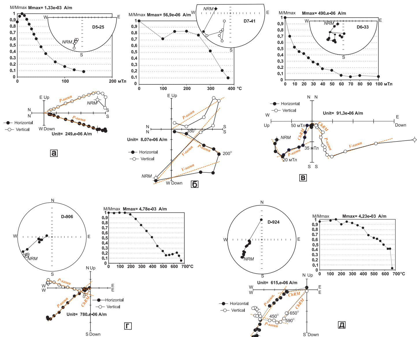
Рис. 3. Примеры ступенчатого размагничивания образцов сероцветных (а, б, в) и красноватых (г, д) пород переменным магнитным полем (а, в) и температурой (б, г, д); на образцах выделены вязкая (V-комн), «пермская» (P-комн) и наиболее стабильная характеристическая (ChRM) компоненты намагниченности.
